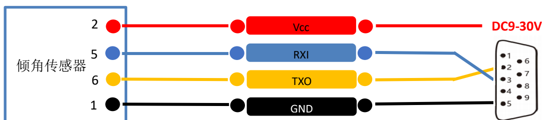
RS232 接线图
